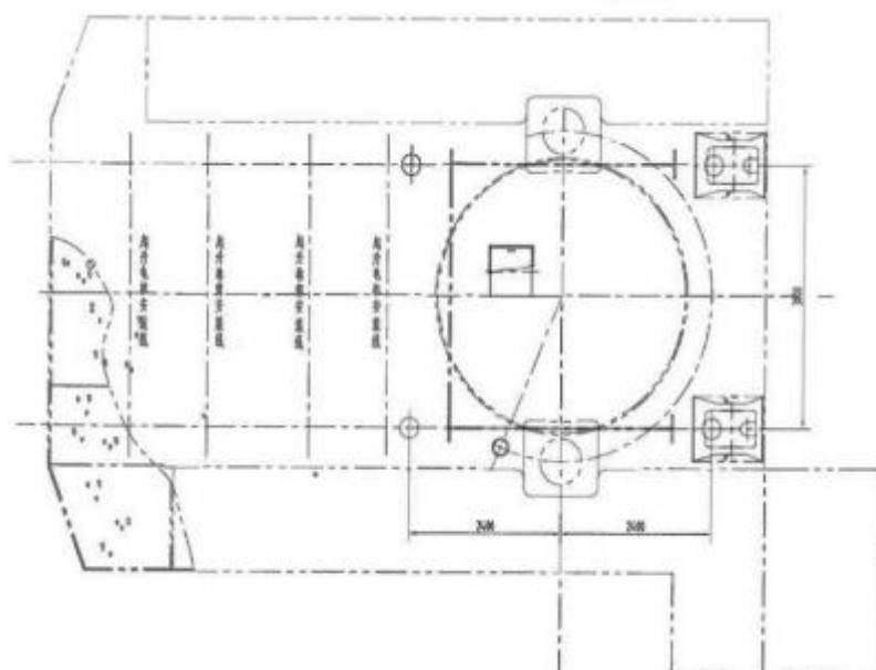
图4 顶升点布置图
