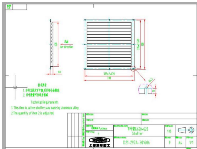
百叶窗 620*620
