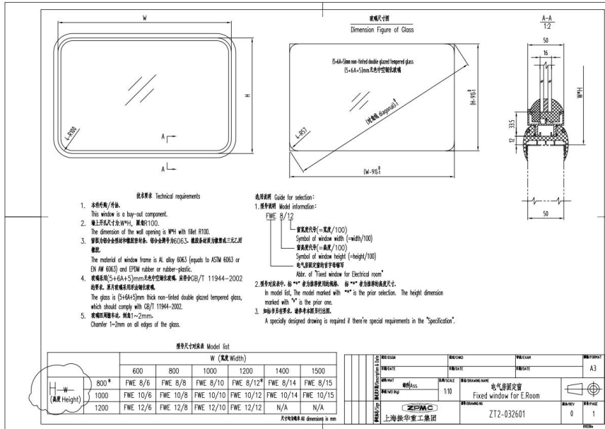
固定窗 ZT2-032601
