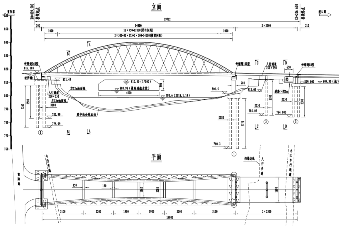
图 1.3-1 云南省怒江渡口大桥桥型布置图
